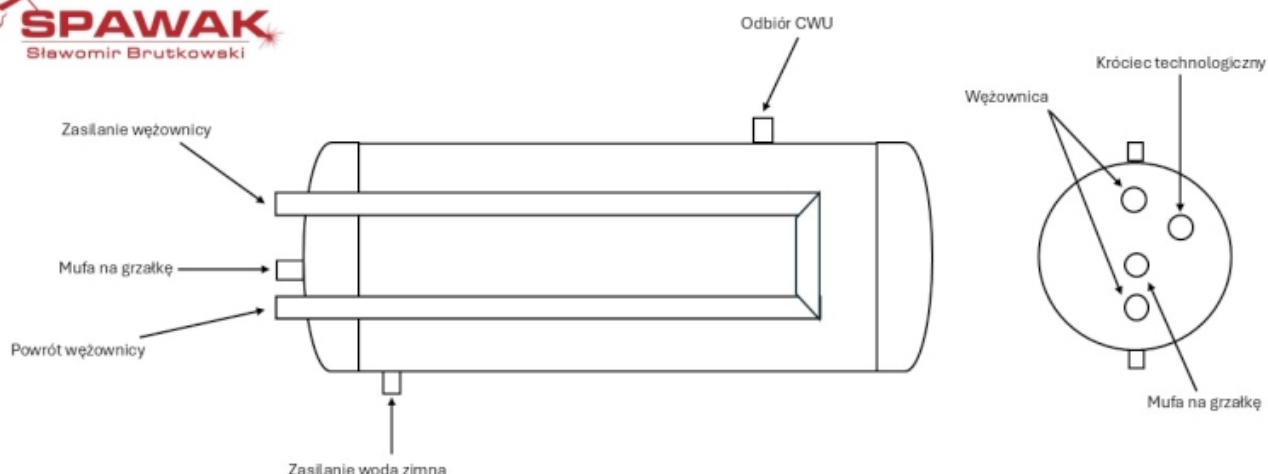
Bojler ze stali nierdzewnej, kwasoodpornej Gat. 316 z jedną pojedynczą węzownicą wzbogaconą.
