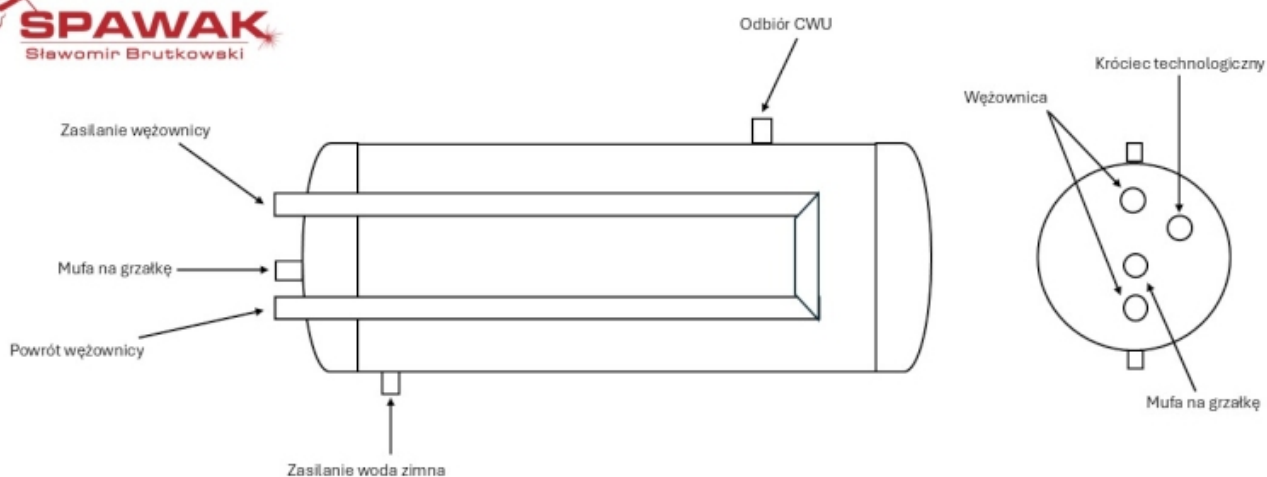
Bojler ze stali nierdzewnej, kwasoodpornej Gat. 316 z jedną pojedynczą węzownicą wzbożoną.
